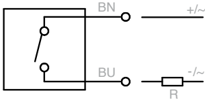
CABLAGGIO - WIRING
